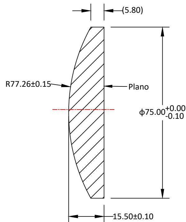
SECTION A-A
