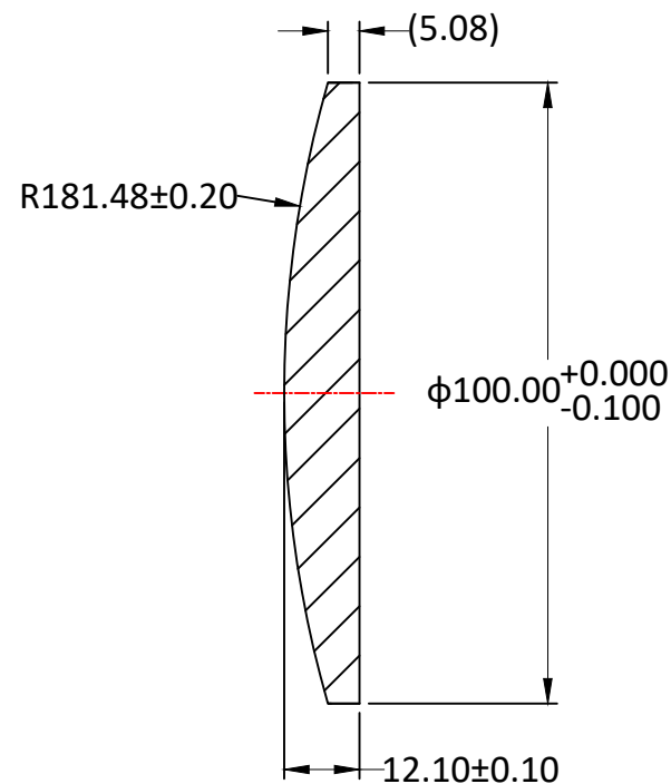
SECTION A-A
