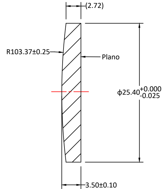
SECTION A-A
