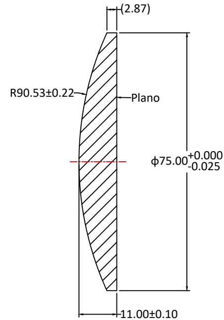
SECTION A-A
