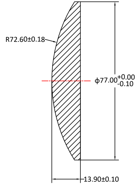
SECTION A-A
